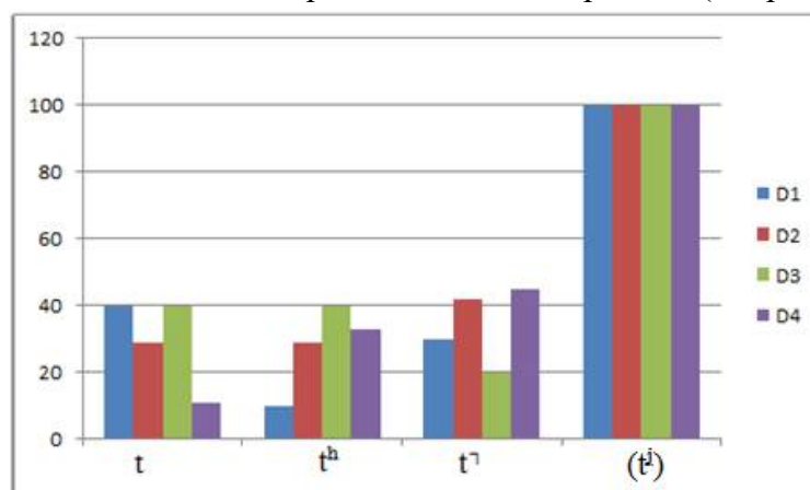
Рис.1. Процент употребления наиболее высокочастотных аллофонов фонем /t/ и /t'/ в позиции конца слова по каждому говорящему
