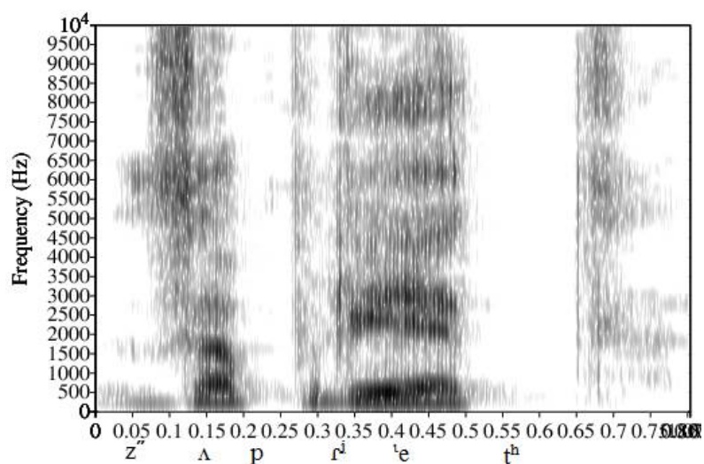
Рис. 3. Реализация слова запрет (D4)
