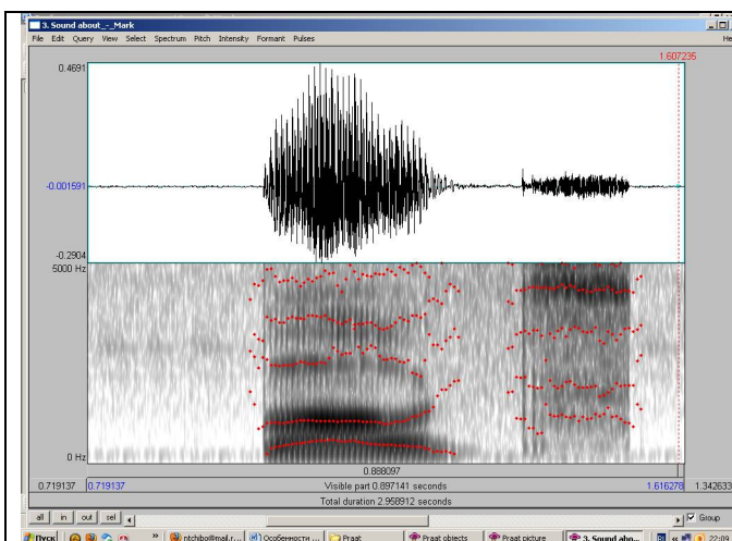
Рис.3. Реализация дифтонга /aʊ/ из слова about . Ядро: F1 – 471, F2 – 1020, глайд: F1 – 489, F2 – 1013
