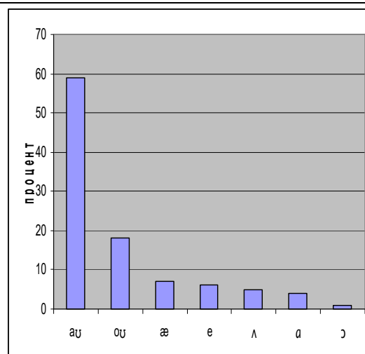
Рис. 4. Перцептивные характеристики дифтонга /aʊ/ в целом по эксперименту.
