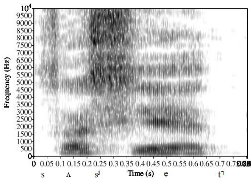
Рис.4. Реализация слова сосед (D4)
