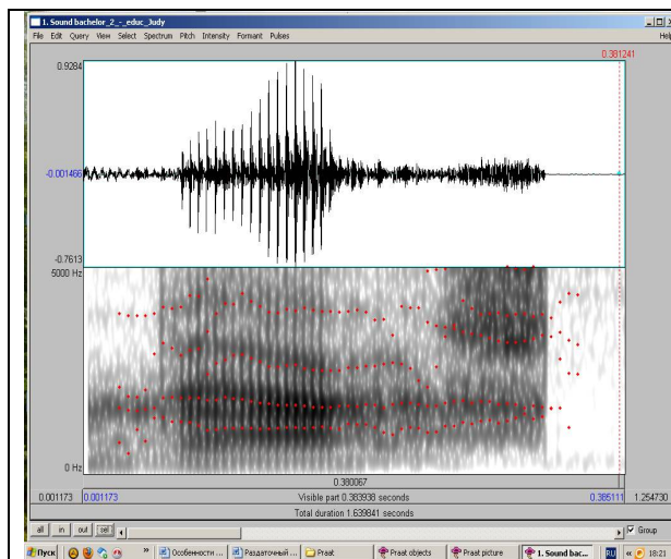
Рис. 1. Спектрограмма стимула bæʃ из слова bachelor , формантные значения F1-F2 = 750 – 1685 Гц, длительность – 111 мс.
