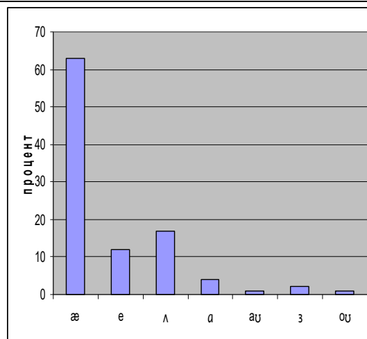
Рис. 2. Перцептивные характеристики монофтонга /æ/ в целом по эксперименту.
