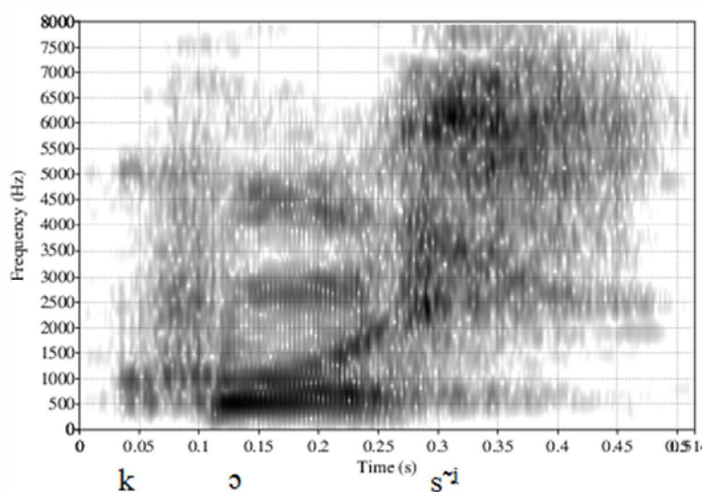
Рис. 2. Реализация слова кость (D1)
